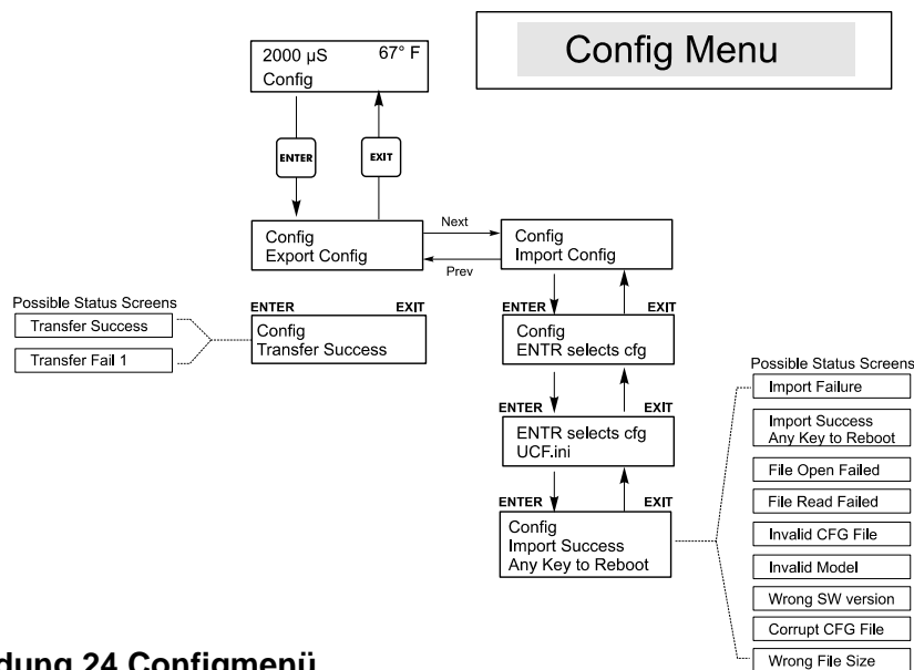
Abbildung 24 Configmenü
