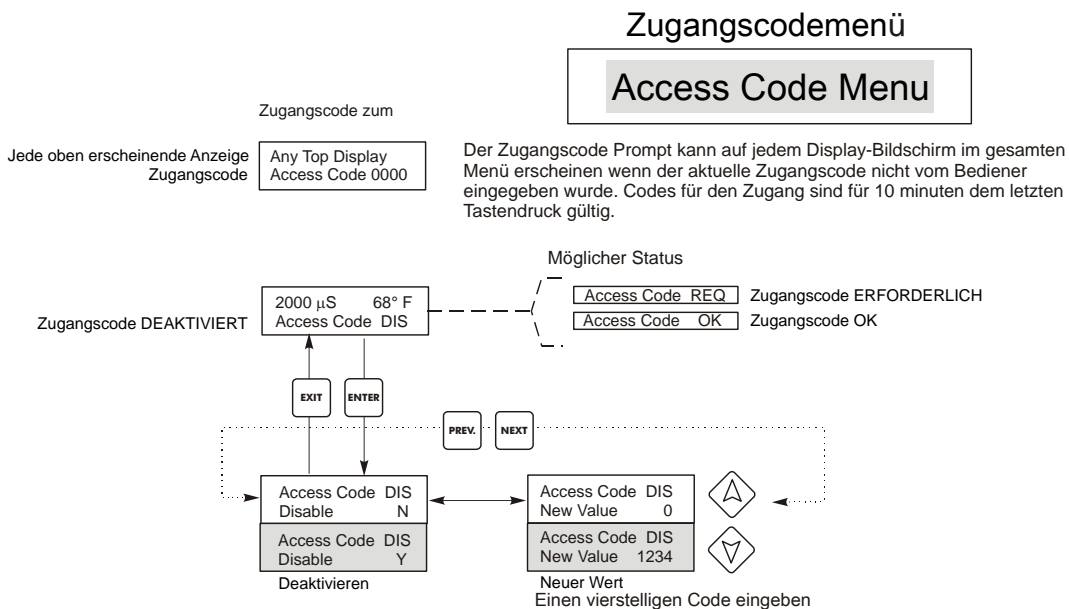
Abbildung 22 Zugangscodemenü
