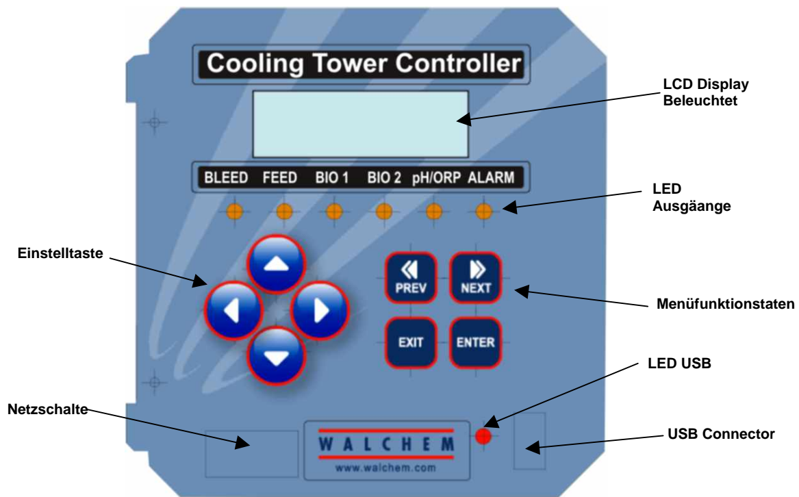
Abbildung 5 Frontplatte
