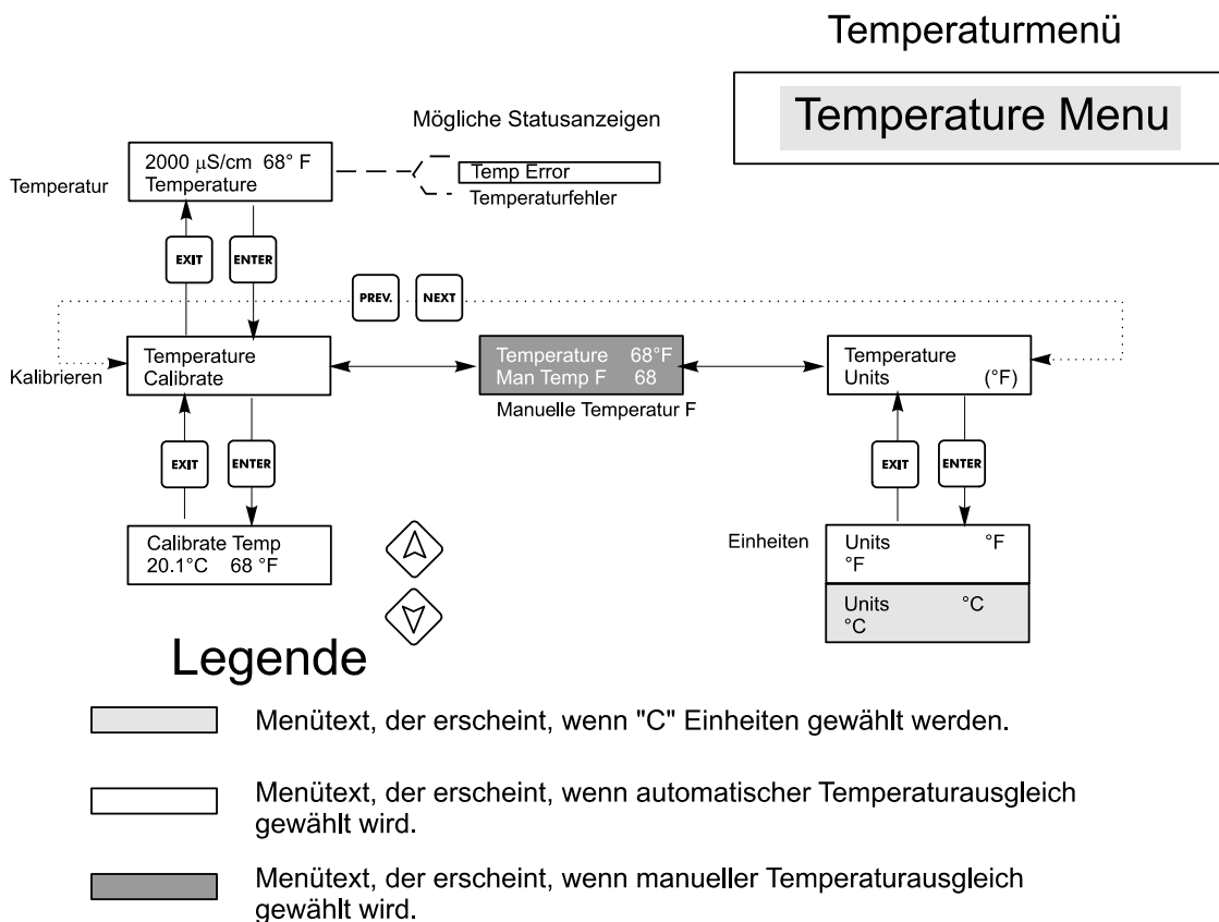
Abbildung 9 Temperaturmenü
